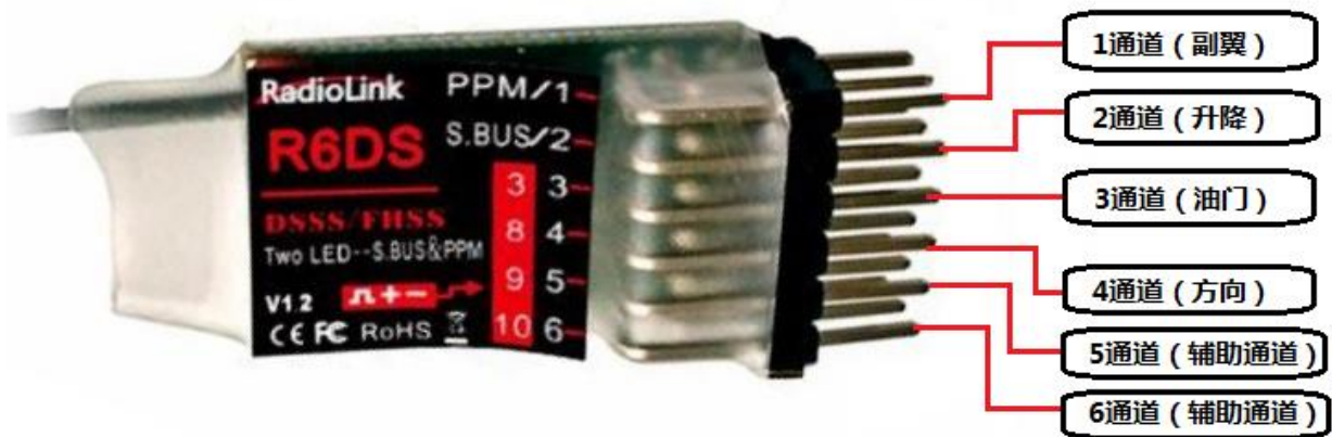
PWM信号工作模式，6通道
